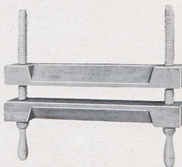
N° 306 PRESSE A TRANCHEFILER
